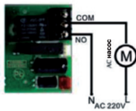
рисунки 3-7 Подключение повысительного насоса
