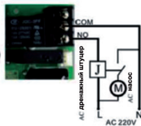
рисунки 3-8 Подключение дренажного штуцера
